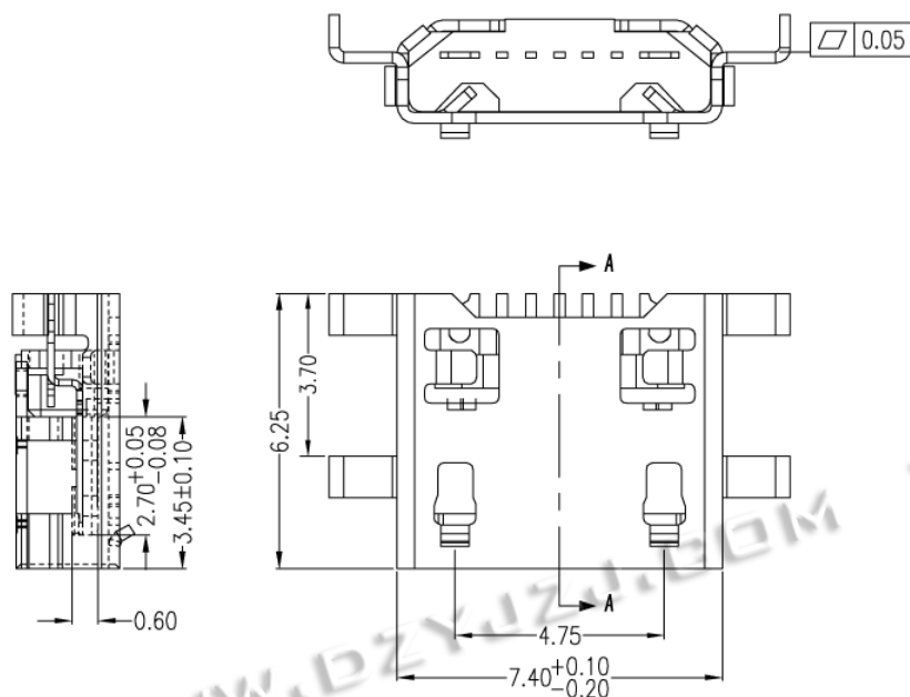
SEC A-A
